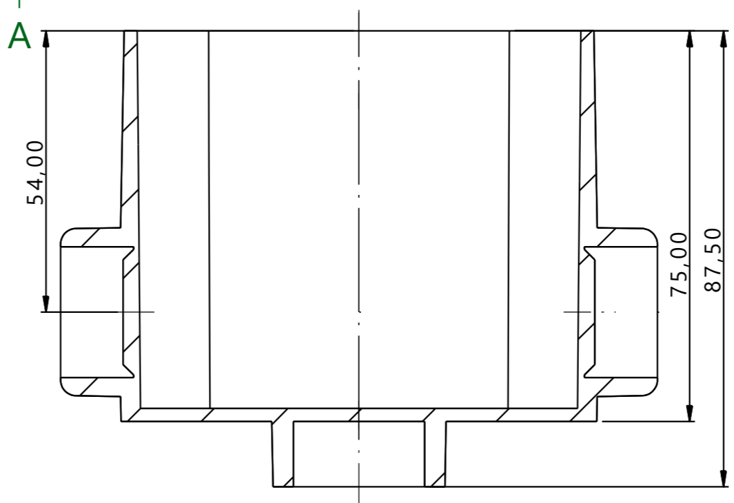
SEÇÃO A-A
